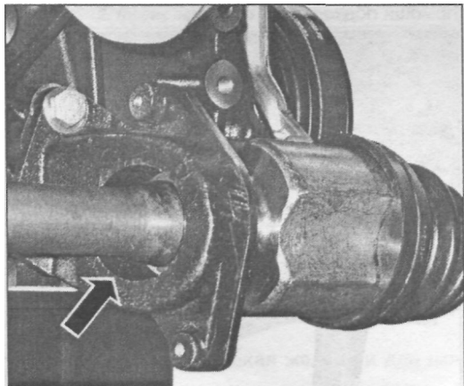
Корпус промежуточного подшипника правой полуоси
