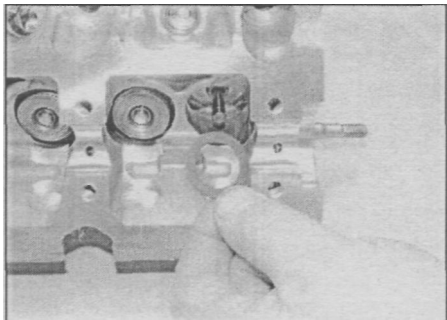
Рис. 10.4,а. Установите седло пружины...
