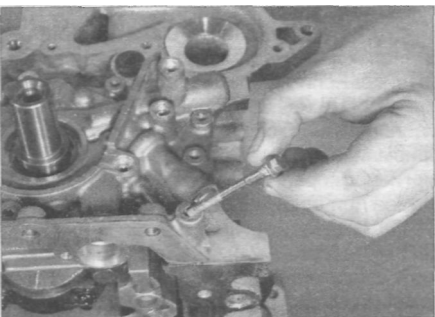
Рис. 14.7. Вывинчивание болтов крепления масляного насоса к блоку цилиндров
