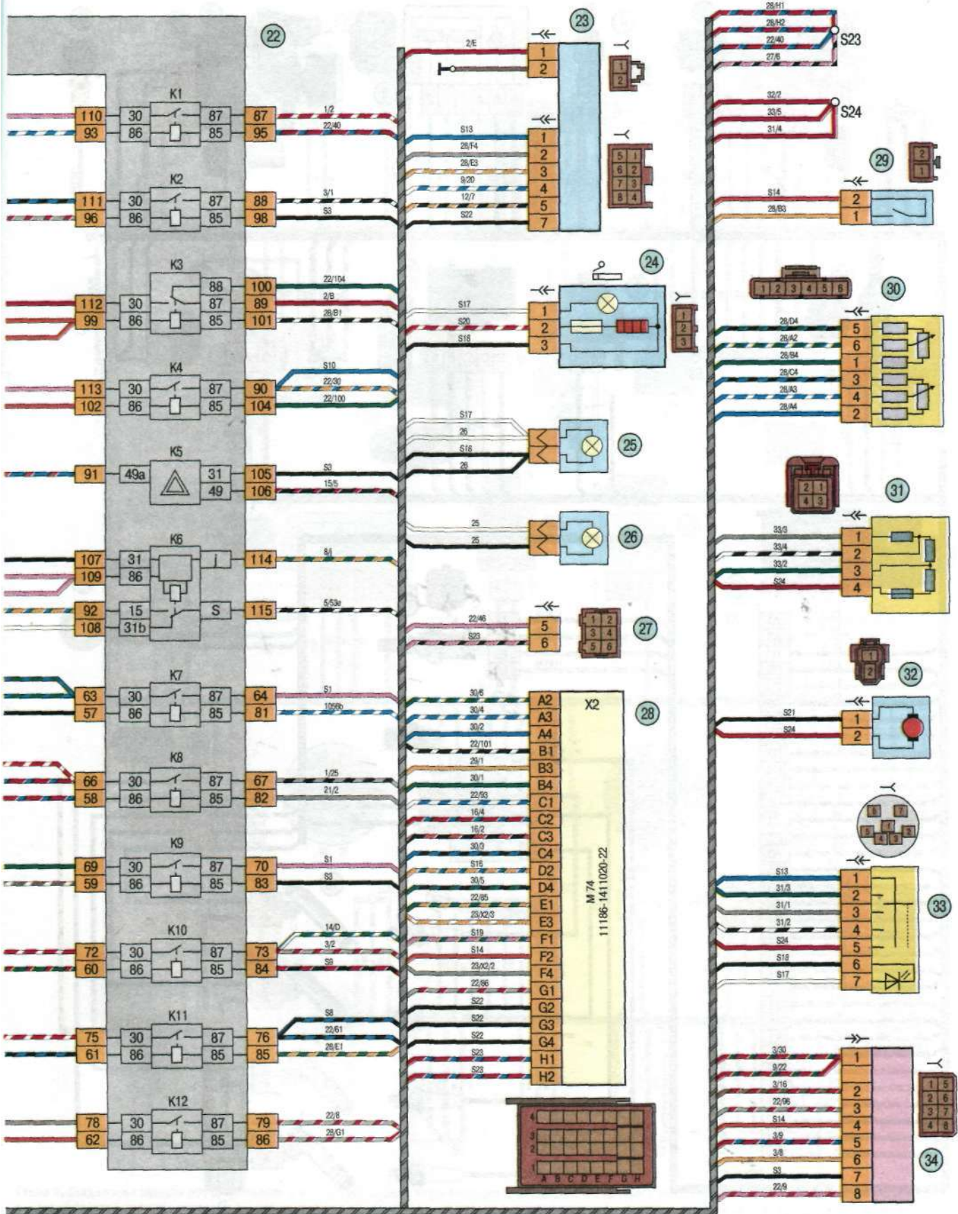
31 – добавочный резистор; 32 – электродвигатель отопителя; 33 – переключатель электродвигателя отопителя; 34 – блок управления системой блокировки дверей; K1 – реле электровентилятора системы охлаждения двигателя; K2 – реле включения блокировки дверей; K3 – дополнительное реле стартера; K4 – дополнительное реле; K5 – реле-прерыватель указателей поворота и аварийной сигнализации; K6 – реле стеклоочистителя; K7 – реле включения дальнего света фар; K8 – реле звукового сигнала; K9 – реле включения ближнего света фар; K10 – реле включения обогрева заднего стекла; K11 – главное реле; K12 – реле топливного насоса
