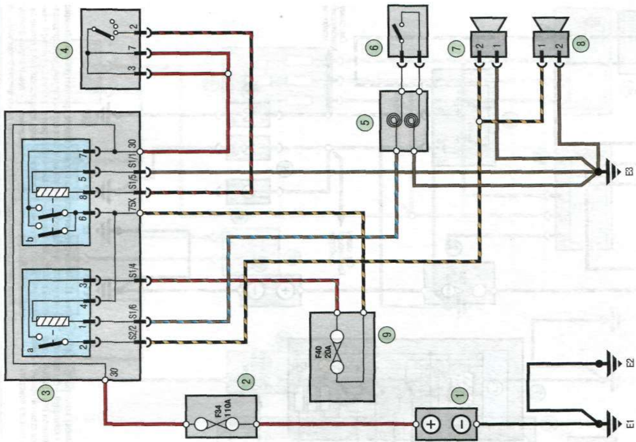
Схема 11. Звуковой сигнал: 1 – аккумуляторная батарея; 2 – монтажный блок плавких перемычек и предохранителей в моторном отсеке; 3 – монтажный блок реле в салоне автомобиля; 4 – выключатель (замок) зажигания; 5 – контактное кольцо; 6 – клавиша звукового сигнала; 7 – сигнал высокого тона; 8 – сигнал низкого тона; 9 – монтажный блок предохранителей в салоне автомобиля
