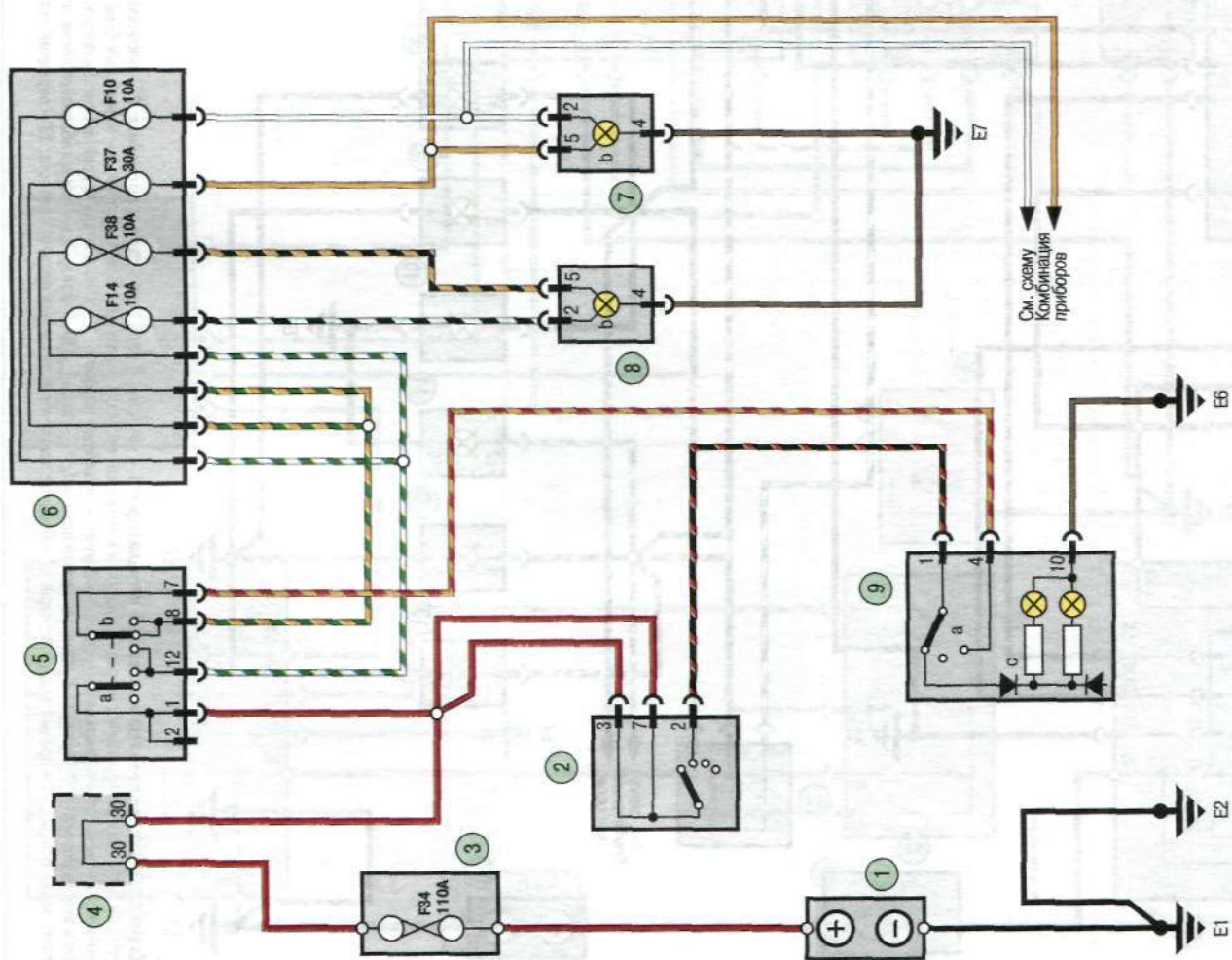
Схема 10. Главное освещение: 1 – аккумуляторная батарея; 2 – монтажный блок плавких перемычек и предохранителей в моторном отсеке; 3 – монтажный блок реле в салоне автомобиля; 4 – рычаг переключателя наружного освещения и указателей поворота; 5 – монтажный блок предохранителей в салоне автомобиля; 6 – правая блок-фара (а – лампа габаритного огня, б – лампа ближнего/дальнего света); 7 – левая блок-фара; 8 – выключатель (замок) зажигания; 9 – комбинация приборов
