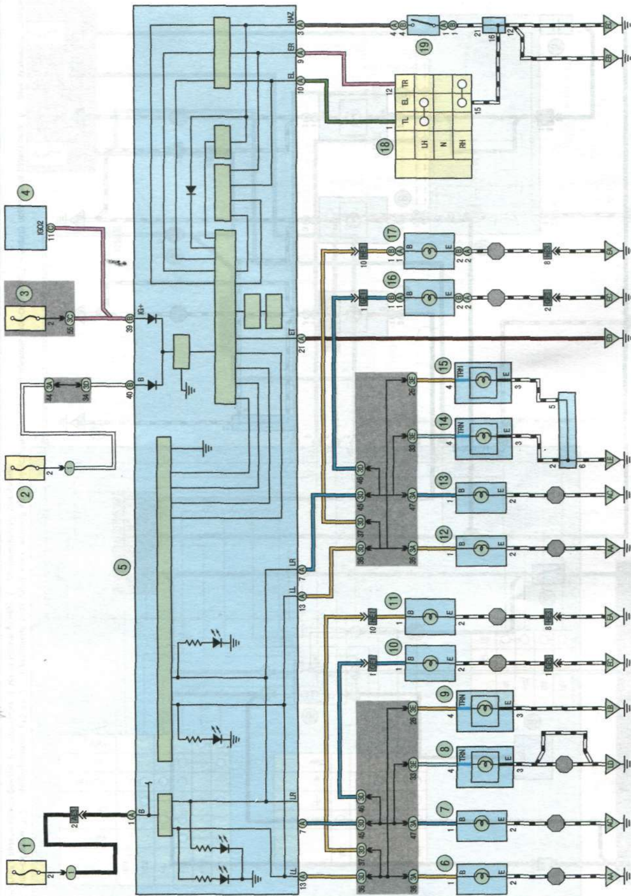
Схема 6. Передние и боковые указатели поворота и аварийная сигнализация (5 А); 4 – предохранитель (10 А); 3 – предохранитель (10 А); 2 – предохранитель (10 А); 1 – указатель поворота в правой блок-фаре (вариант 1); 7 – указатель поворота в левом наружном зеркале заднего вида (вариант 1); 11 – указатель поворота в левом блоке фары (вариант 1); 12 – указатель поворота в правой блок-фаре (вариант 2); 13 – указатель поворота в левом блоке фары (вариант 2); 14, 15 – контрольные лампы в комбинации приборов (вариант 2); 16 – боковой указатель поворота в левом наружном зеркале заднего вида (вариант 2); 17 – указатель поворота в левом наружном зеркале заднего вида (вариант 2); 18 – подрулевой переключатель наружного освещения и указателей поворота; 19 – выключатель аварийной сигнализации
